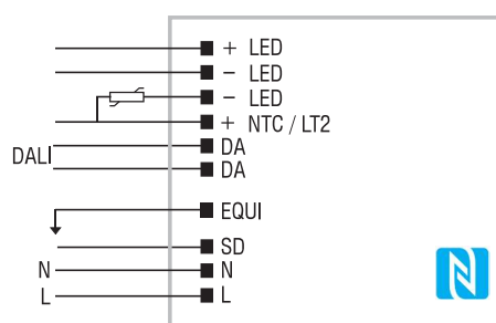
WIRELESS PROGRAMMING diagram Collegamento per PROGRAMMAZIONE WIRELESS
