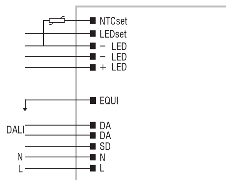
DALI / MIDNIGHT / BILEVEL diagram for 165W Collegamento DALI / MIDNIGHT / BILEVEL per 165W
