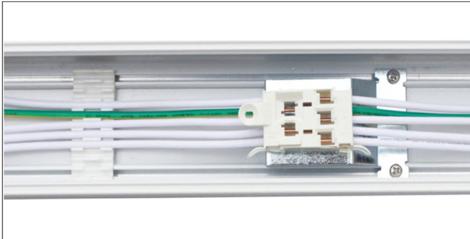
5-vodičová lišta
