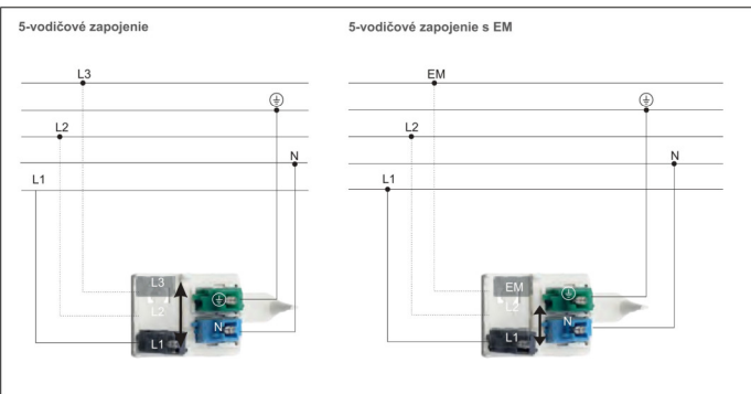
5-vodičová lišta
