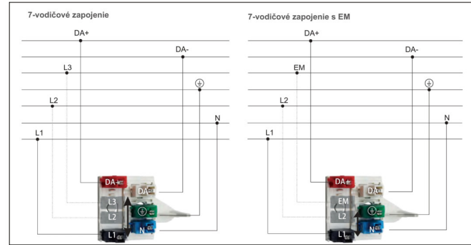
7-vodičová lišta
