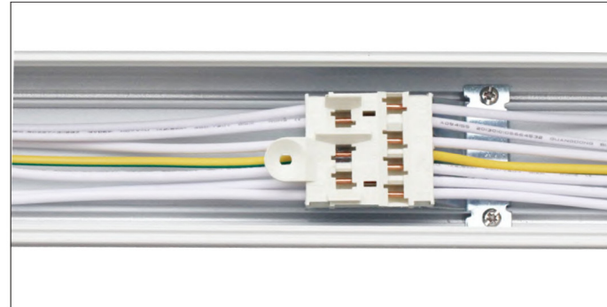
7-vodičová lišta
